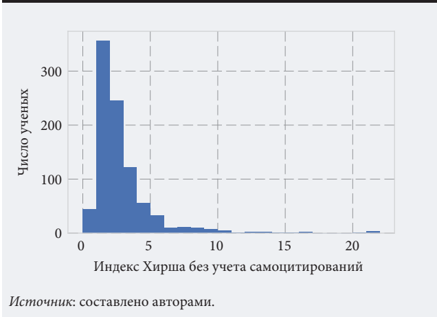
Рис. 7. Гистограмма распределения индекса Хирша без учета самоцитирований
